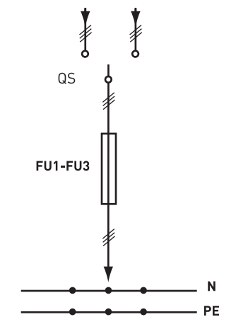
Рис. 3 Принципиальная электрическая схема ЯРП-XXX-XX-П УХЛЗ
